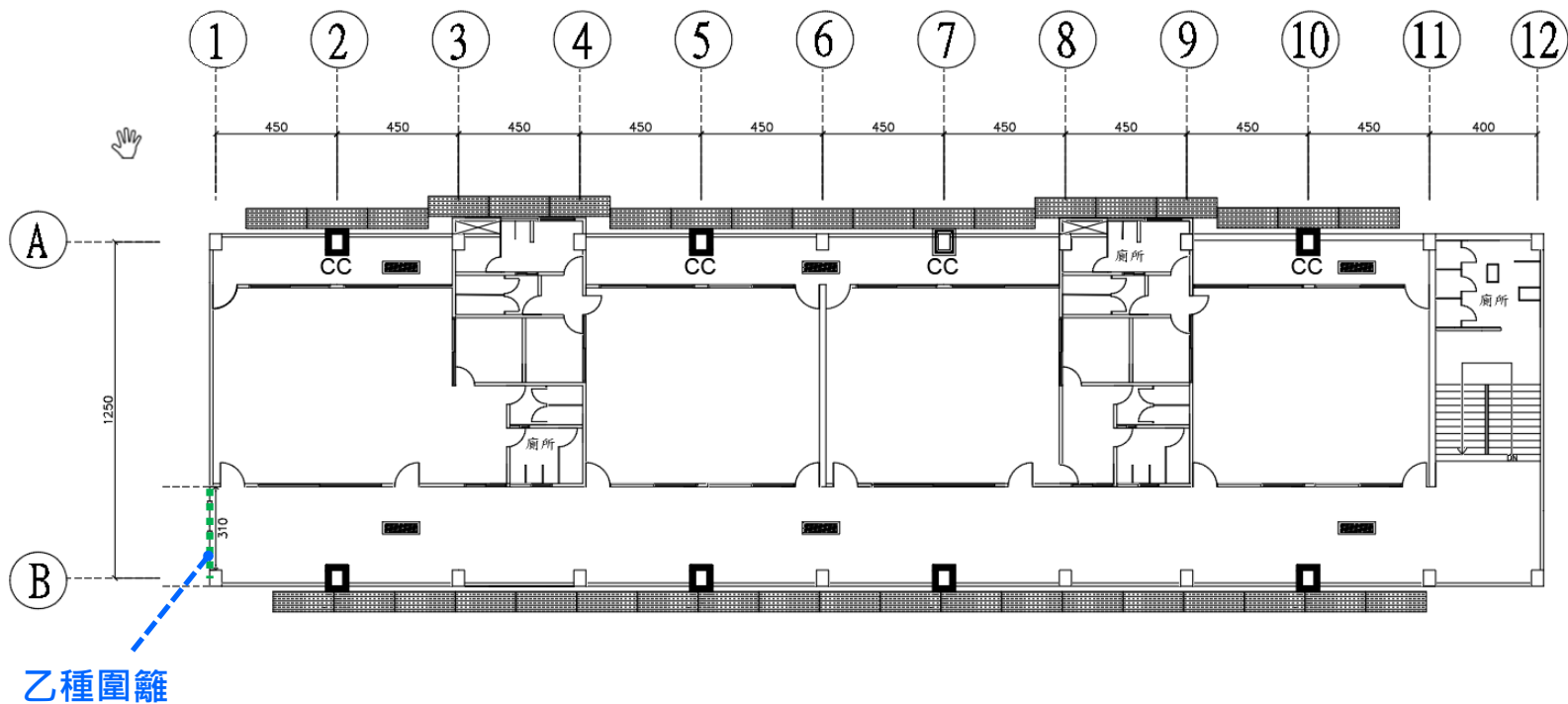
假設工程二樓建築平面圖
