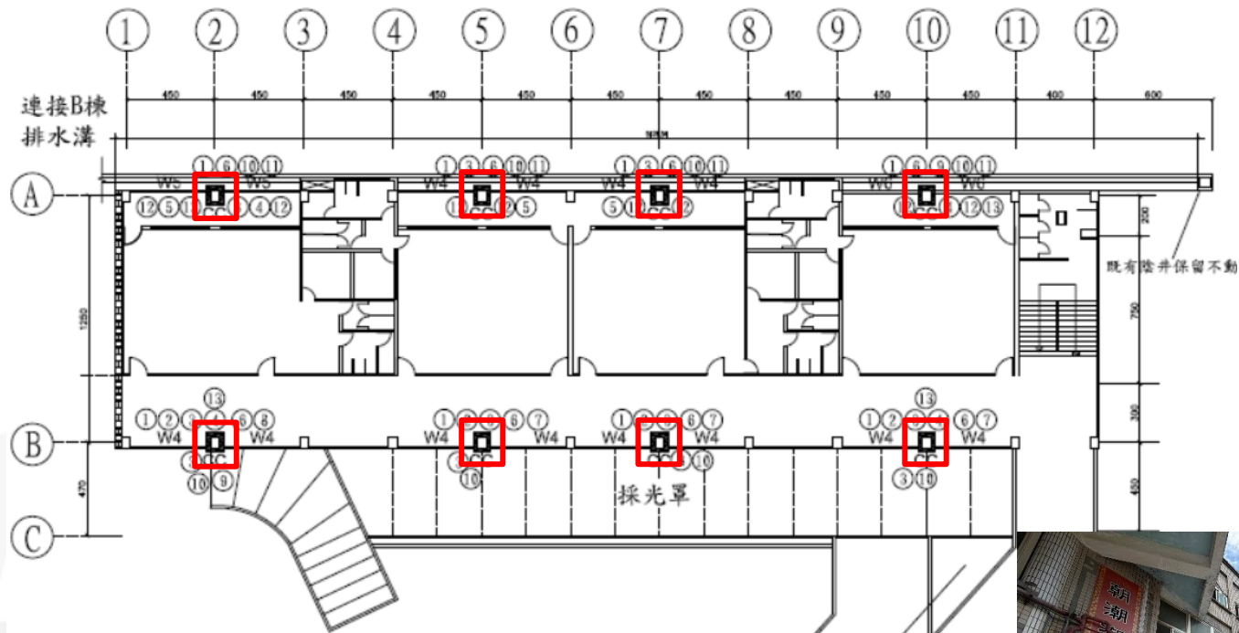
補強後一樓平面圖(A棟)
