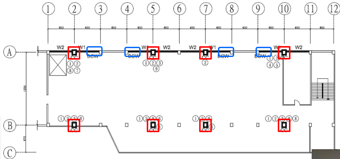
補強後地下一樓平面圖(A棟)
