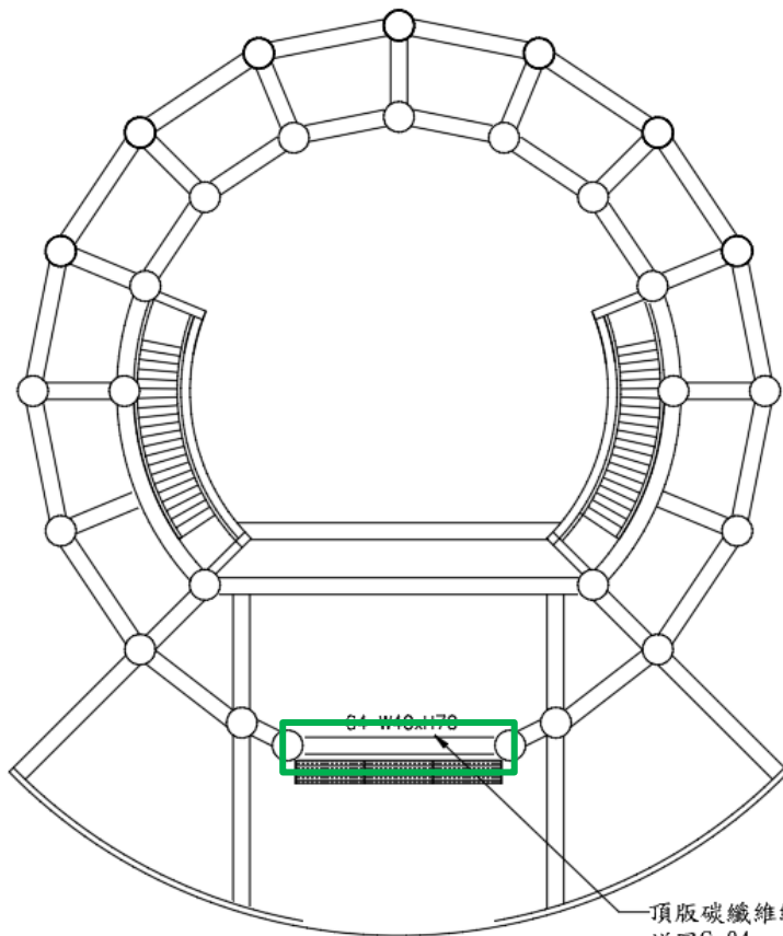
B棟補強後三樓修復平面圖
