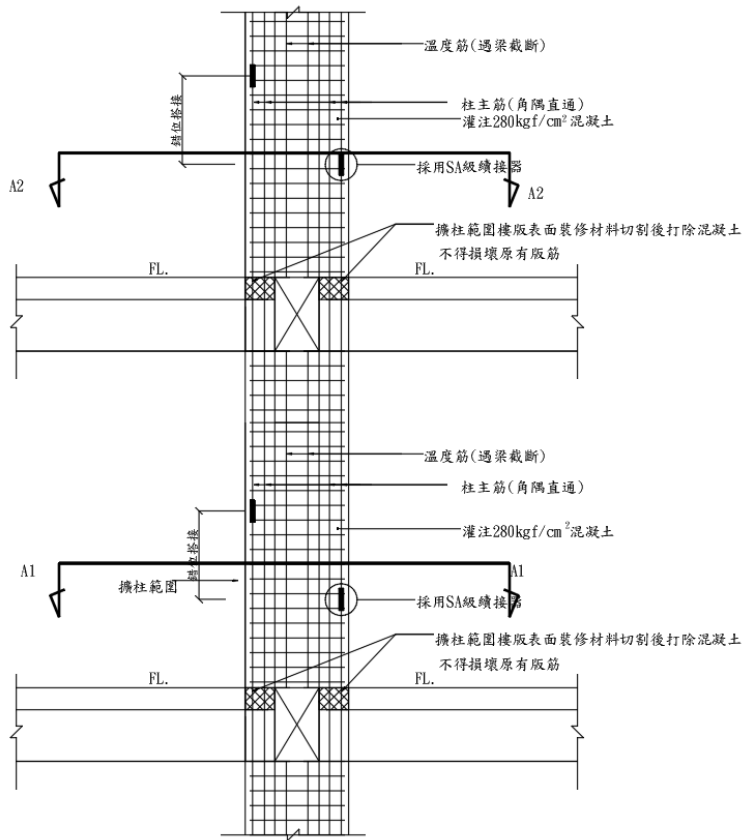
擴柱施工圖
